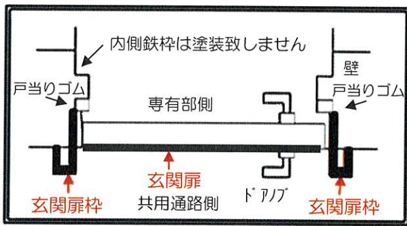
玄関扉枠塗装箇所断面図
